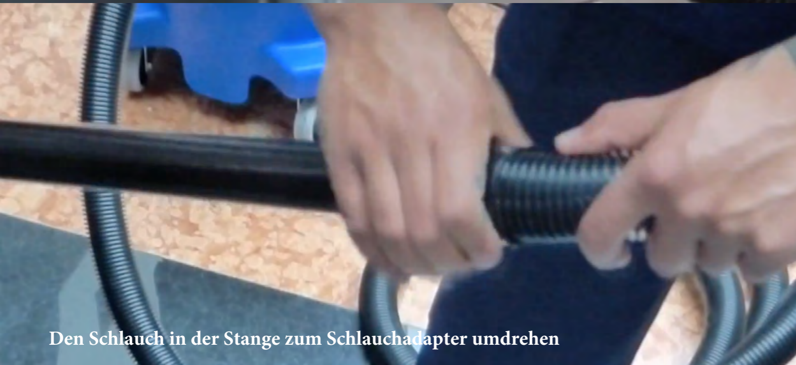
Schließen Sie den Schlauch an den Sauger an
